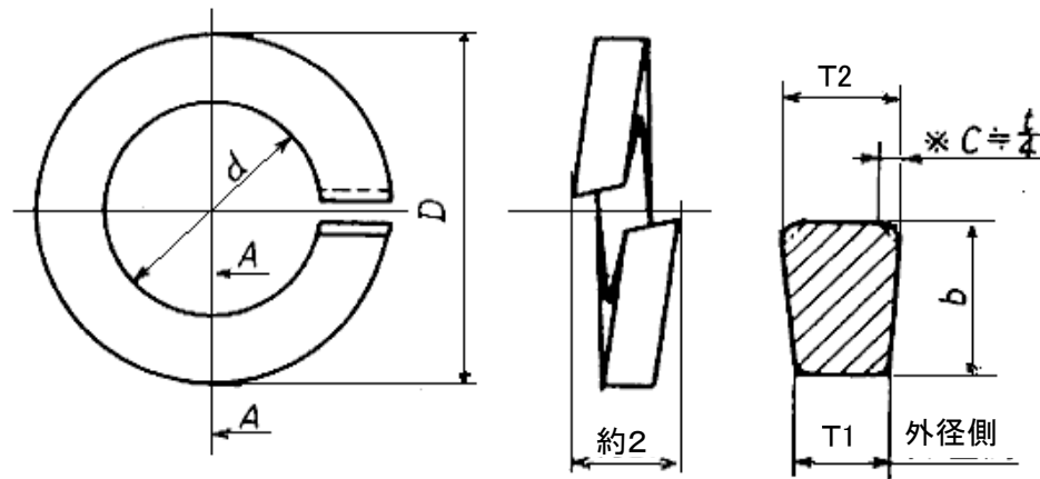
断面 A-A
